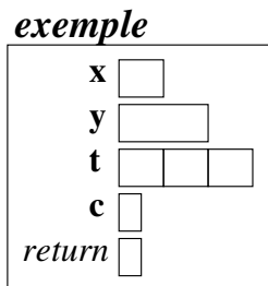
FIGURE 7.1 – Zone de mémoire occupée par la fonction exemple
