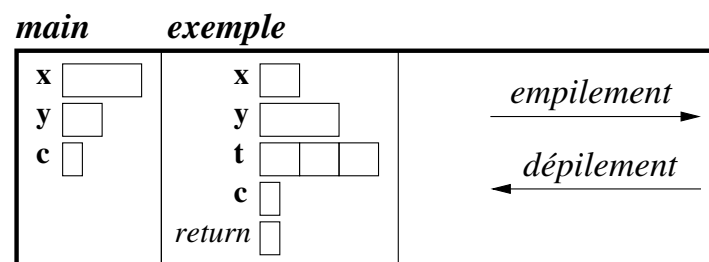
FIGURE 7.2 – La pile pendant l'appel de fonction exemple
