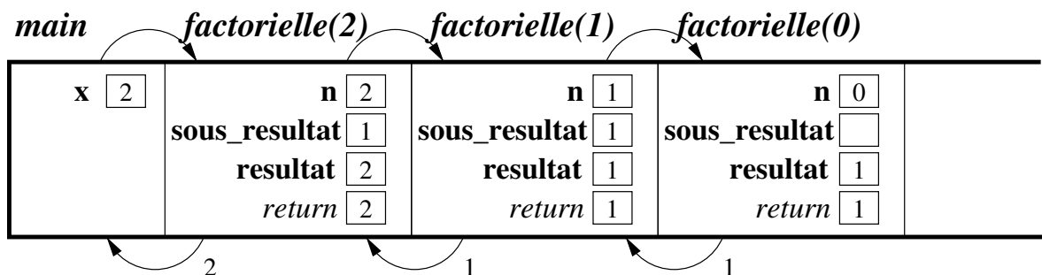
FIGURE 7.3 – Enchaînement des appels récursifs pour factorielle(2)
